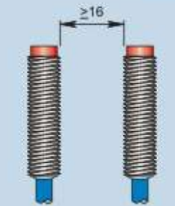
Montaggio affiancato
