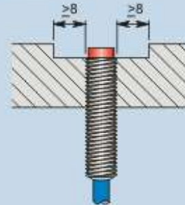
Montaggio sporgente
